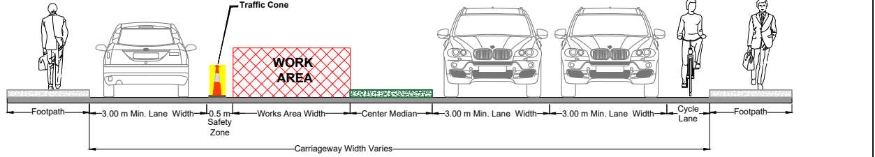
SECTION A-A
