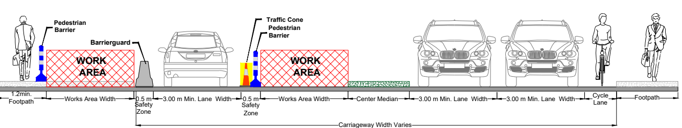
SECTION A-A
